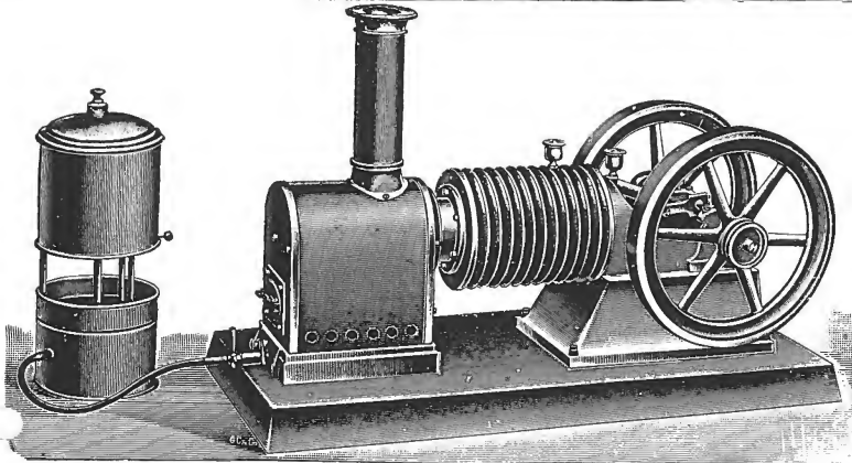
No. 84. Heete lucht motor met extra spiritus-generator, zeer sterk Prijs f 45.—
