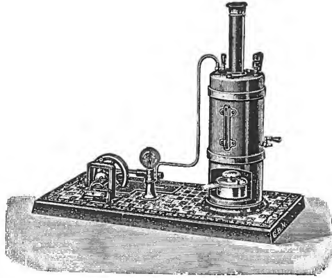
No. 50. Locomobile met oscileerende cilinder, de machine kan naar verkiezing al of niet aan de dynamo gekoppeld worden, deze dynamo doet een lampje van 4 volt gloeien. . Prijs f 15
